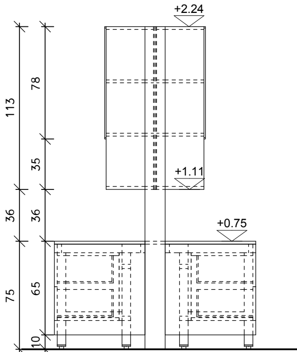
צד
