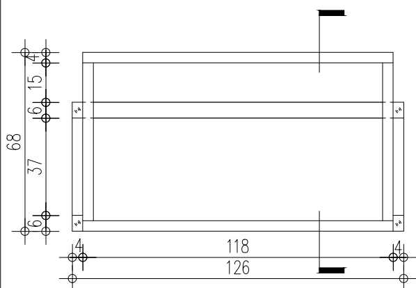
תכנית 1:20
