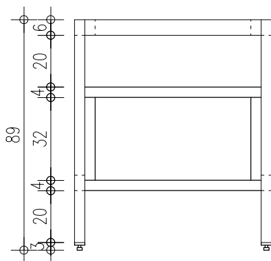
חזית 1:20
