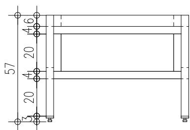
חזית 1:20
