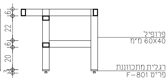
חתך 1:20
