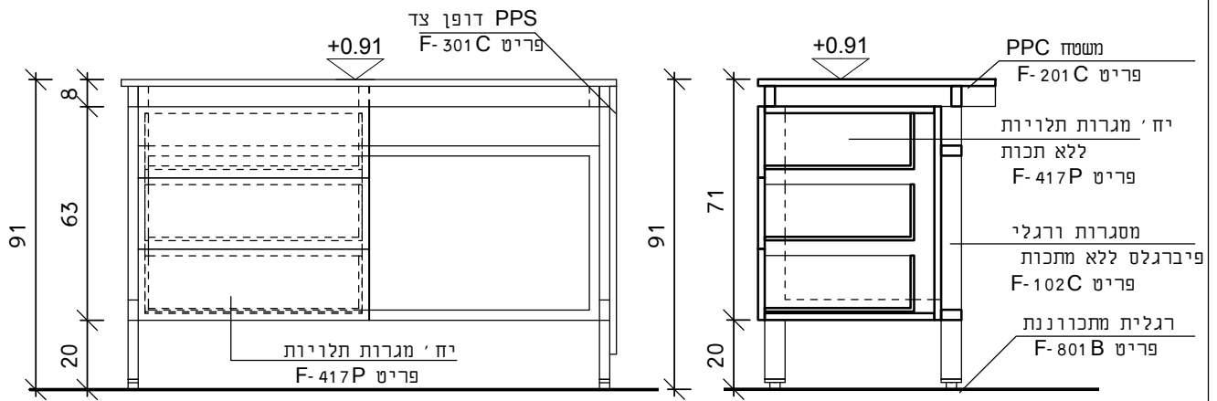
חזית
