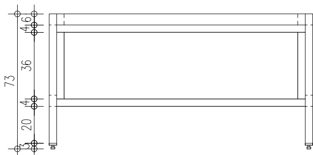
חזית 1:20
