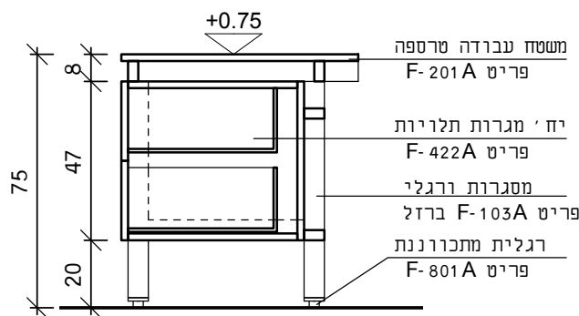
חזית
