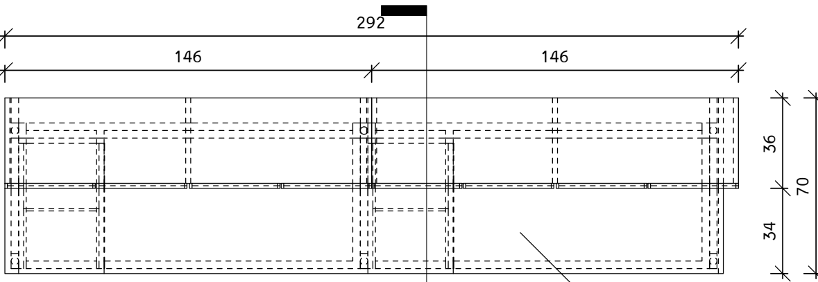
תכנית
