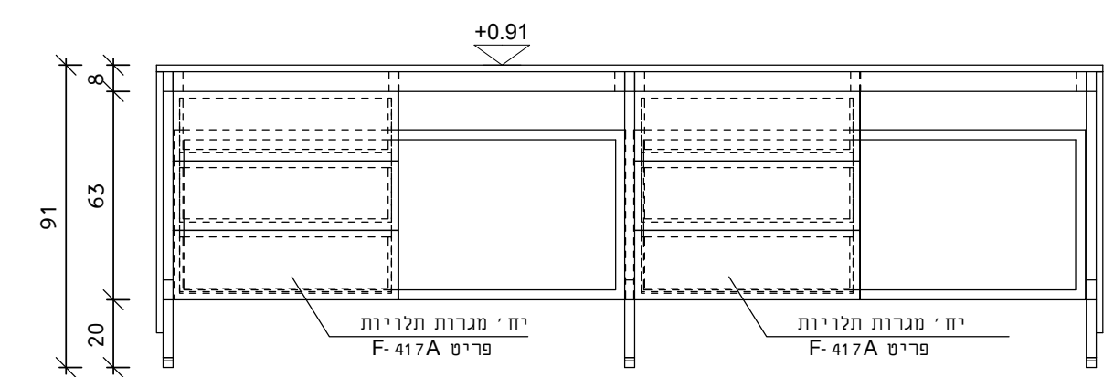
חזית
