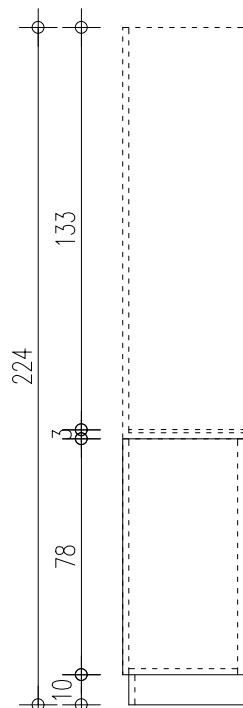
חזית 1:20
