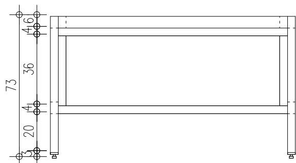
חזית 1:20
