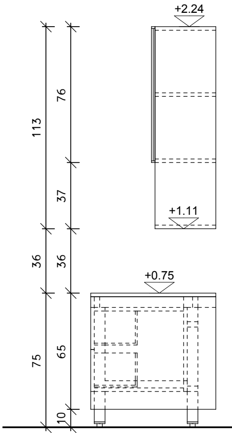
צד
