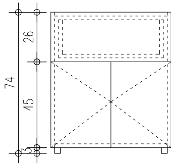
חזית 1:20
