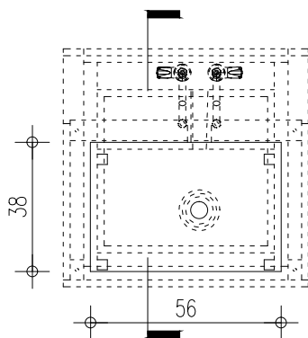
תכנית 1:20
