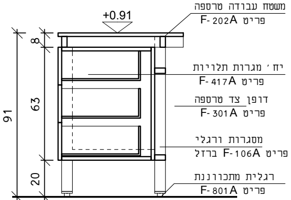
חיתך
