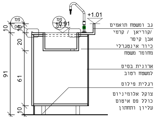
חזית
