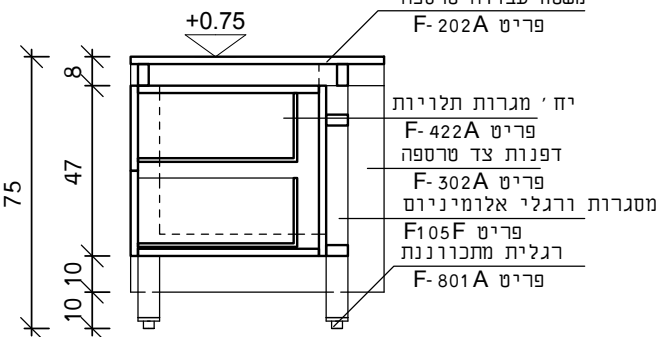
חתך
