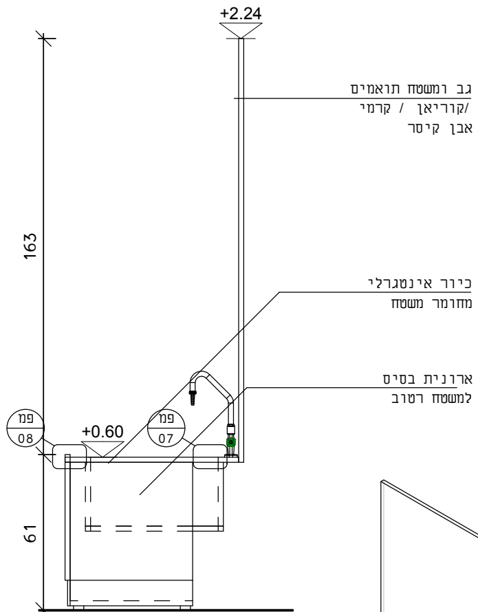
חתר
