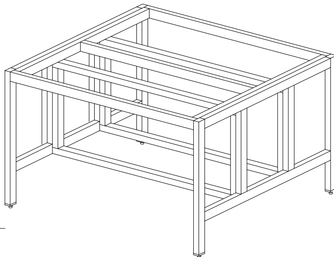
מבט איזומטרי
