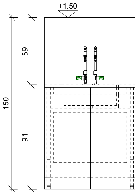
חזית
