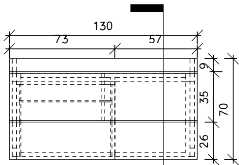
תכנית
