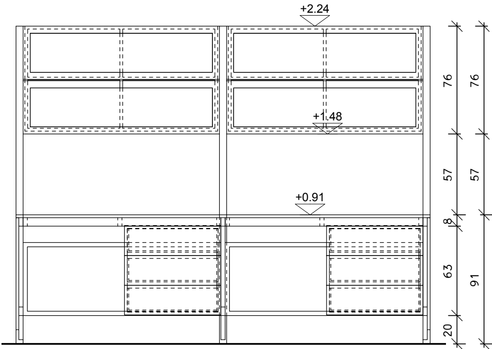
חזית
