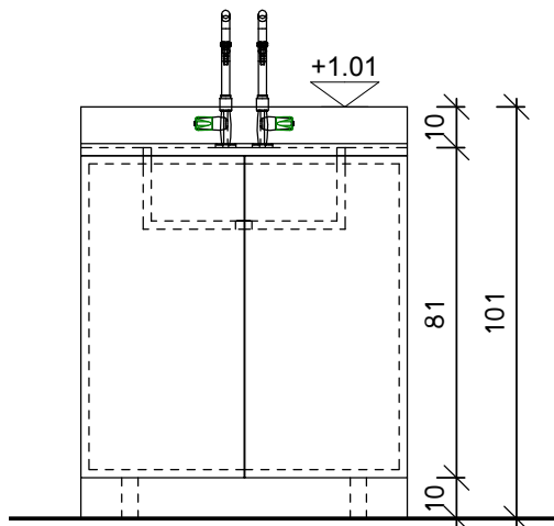
חזית
