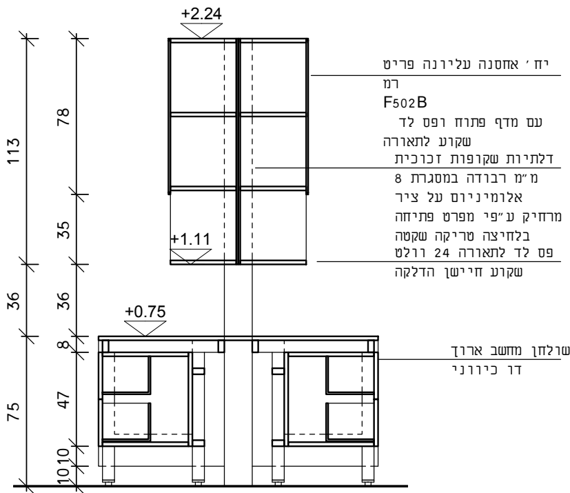
חזית
