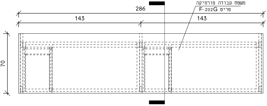
תכנית
