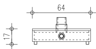
חזית צד 1:20
