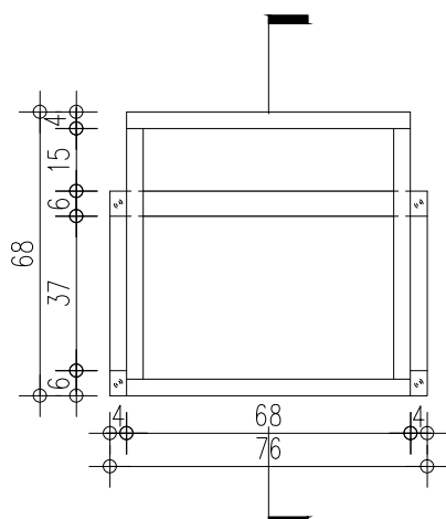
תכנית 1:20
