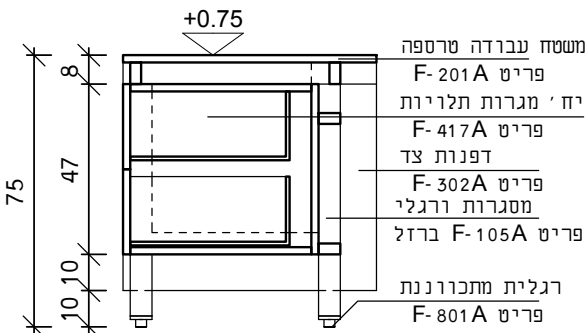
חתך
