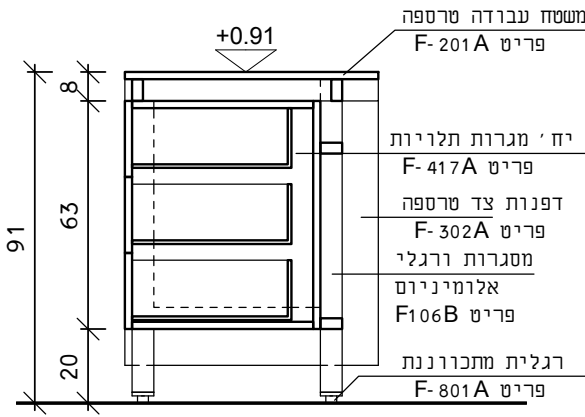
חתך
