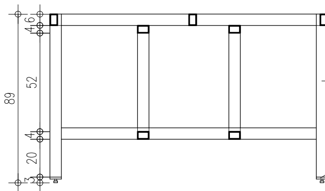
דופן צד
