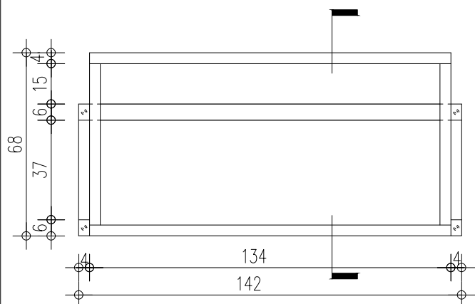
תכנית 1:20
