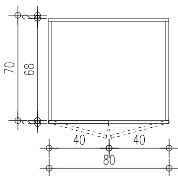
תכנית 1:20
