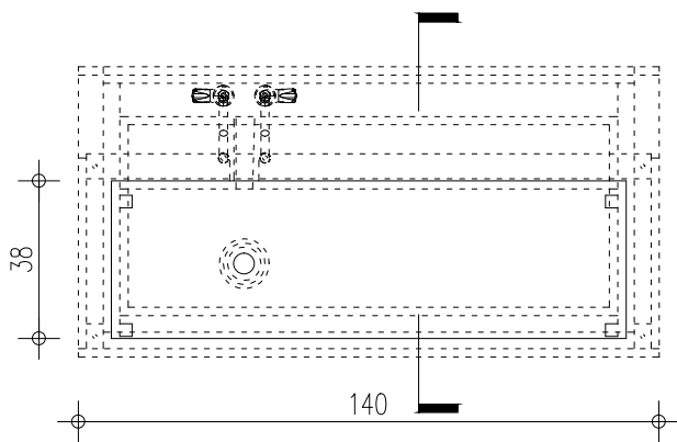
תכנית 1:20
