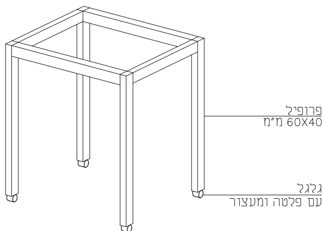
מבט איזומטרי
