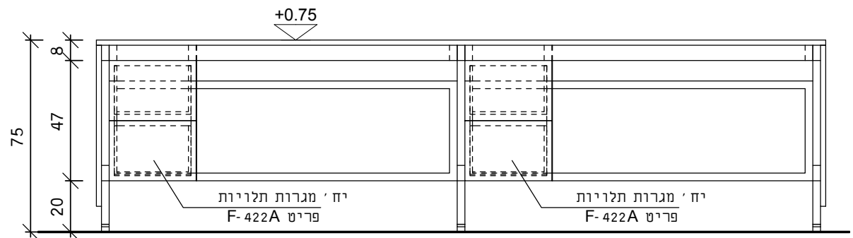
חזית
