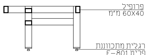
דופן צד 1:20
