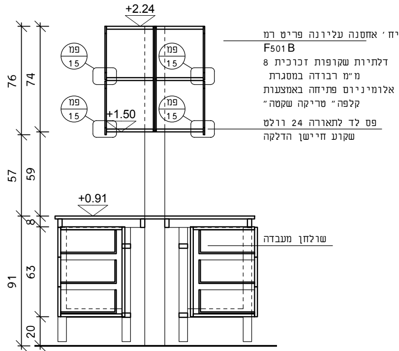
חתר
