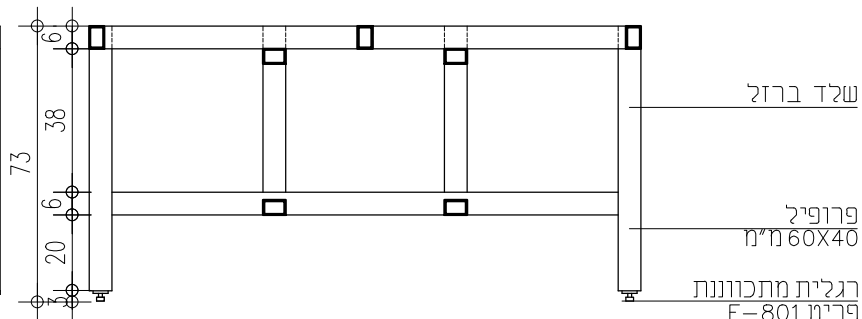
חותך 1:20
