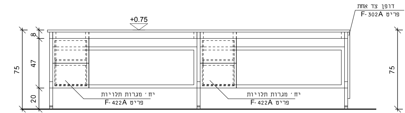
חזית
