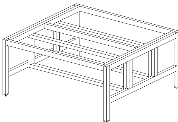
מבט איזומטרי
