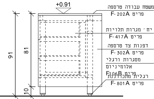
צד
