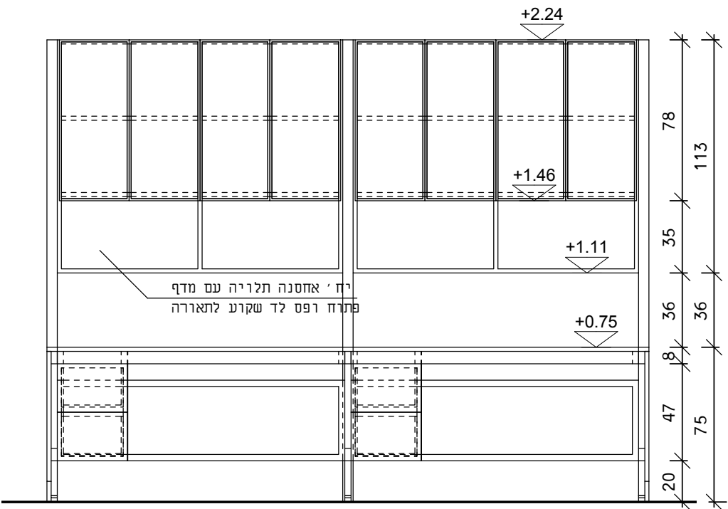
חזית
