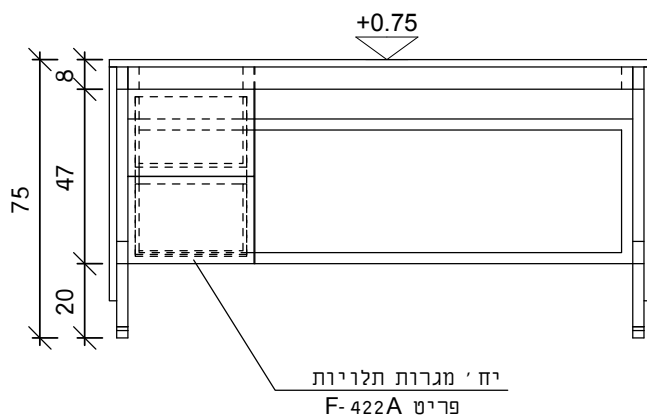
חזית
