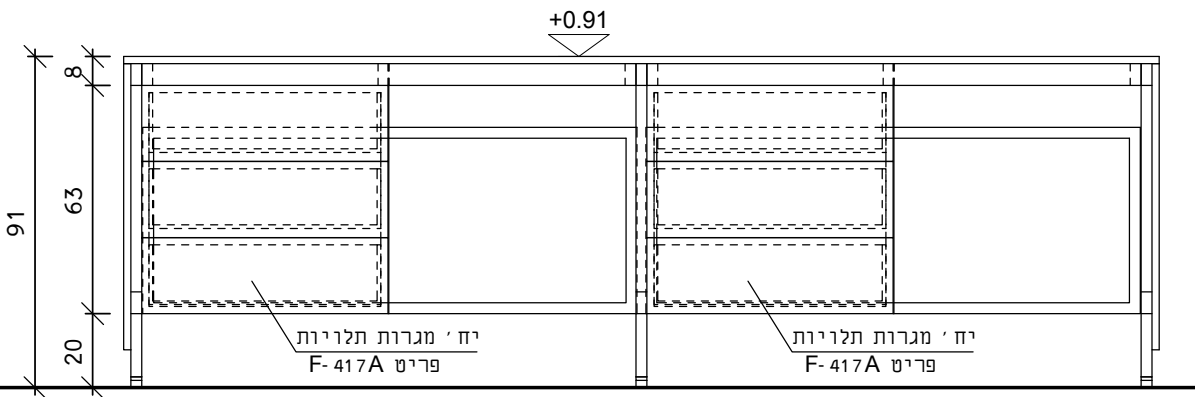
חזית
