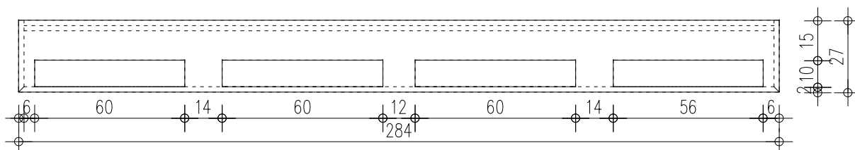
תכנית
