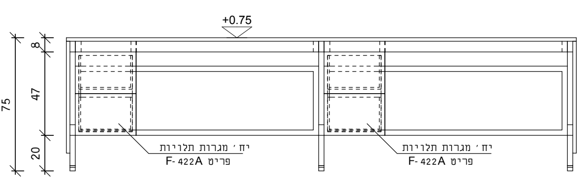
חזית
