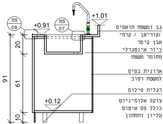
חתך
