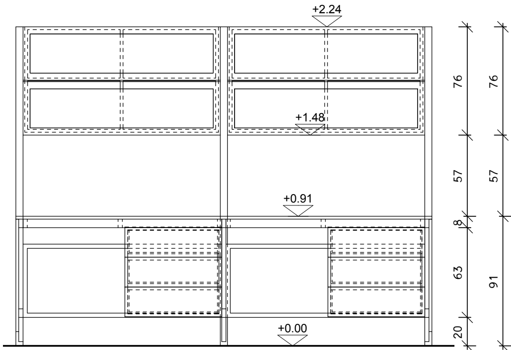
חזית
