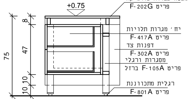
חזית
