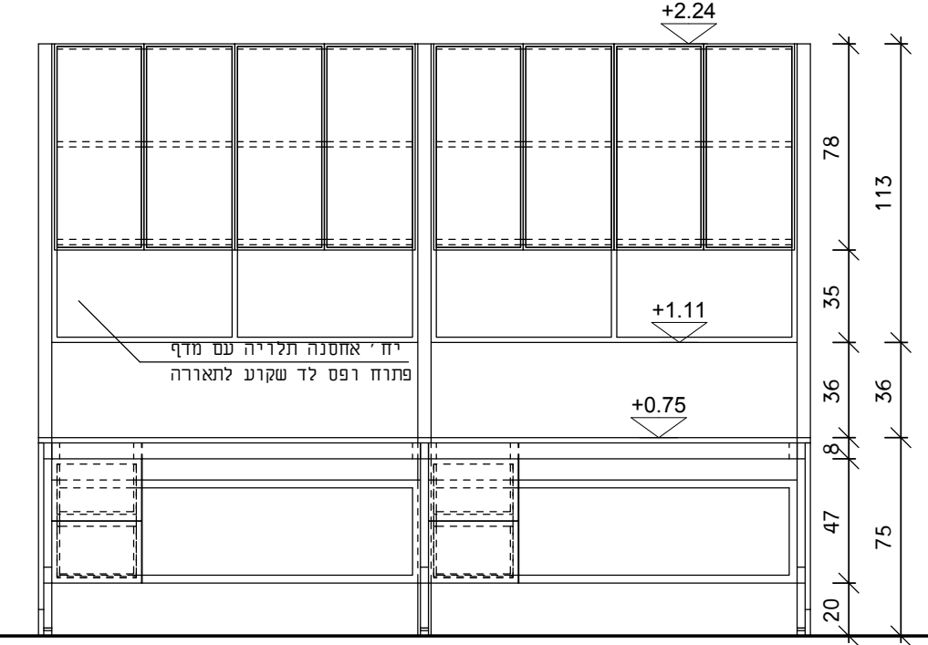
חזית
