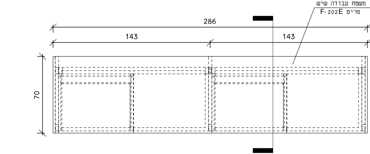
תכנית
