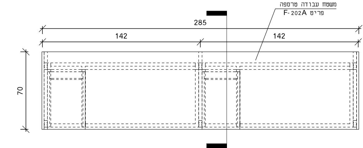
תכנית
