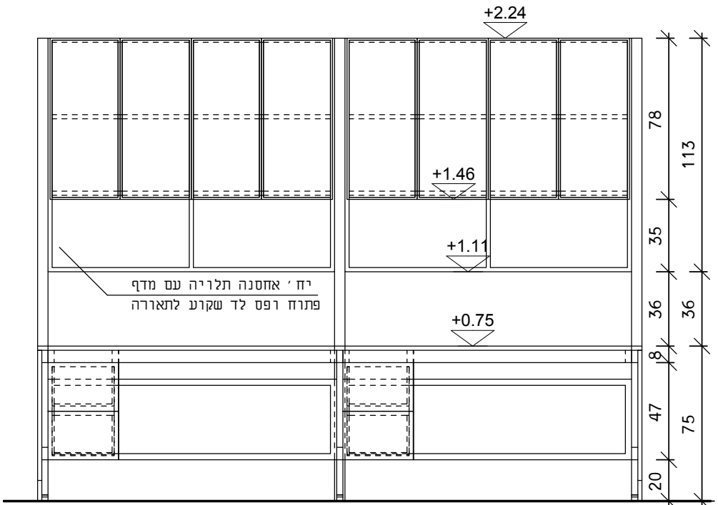
חזית
