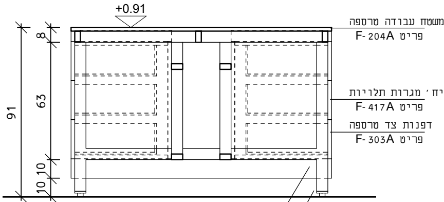
חזית
