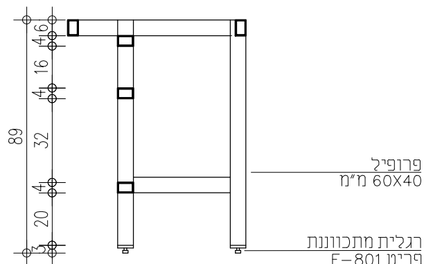
חתך 1:20
