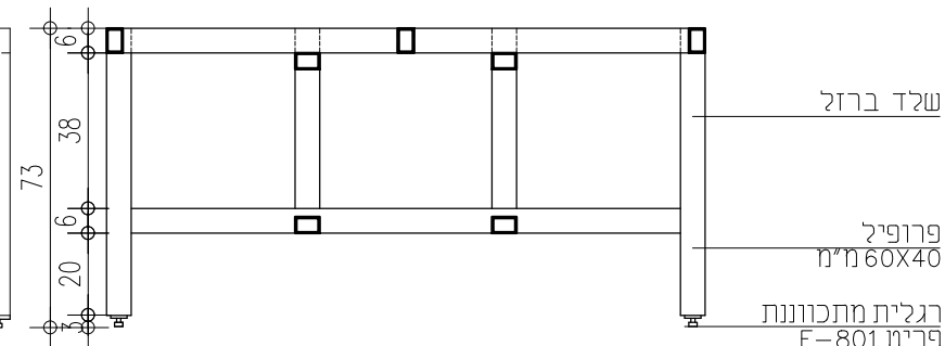
חותך 1:20
