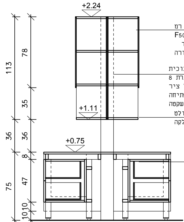
חזית
