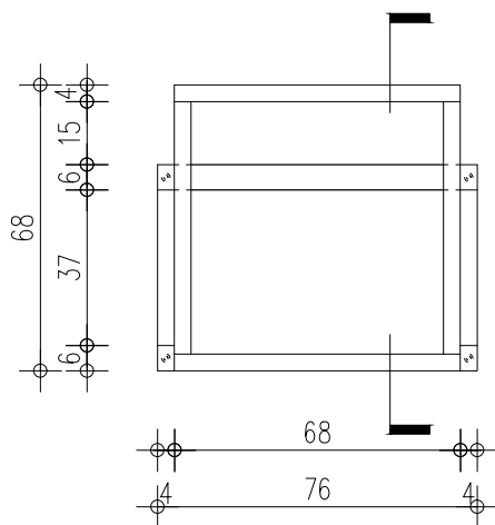
תכנית 1:20
