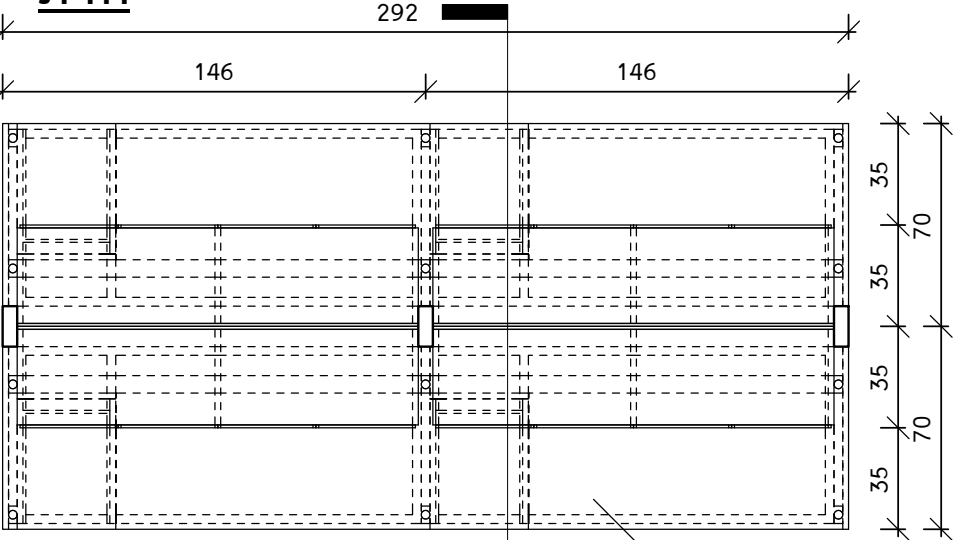
תכנית
