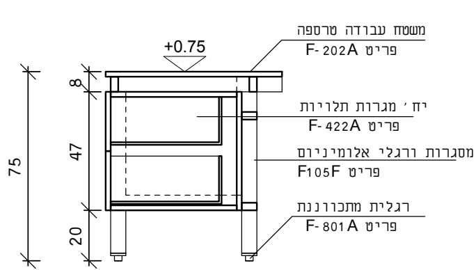
חזית
