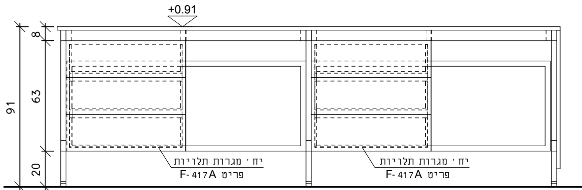
חזית
