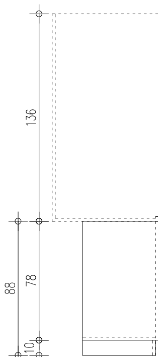
דופן 1:20
