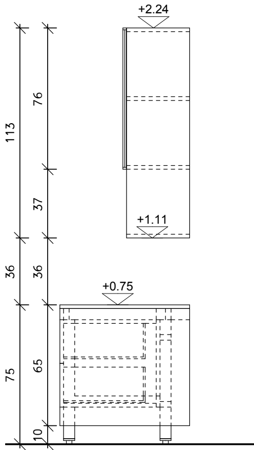
צד
