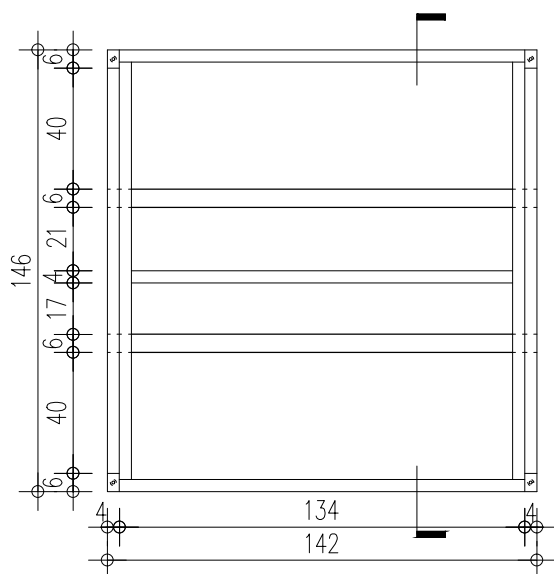
תכנית 1:20
