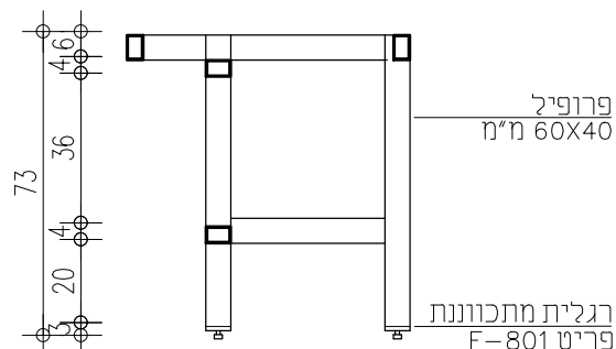
1:20 חתך
