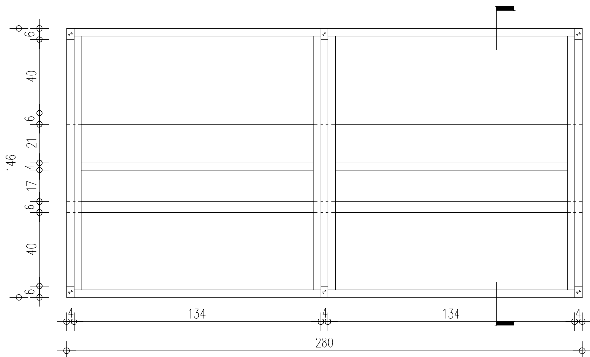
תכנית 1:20
