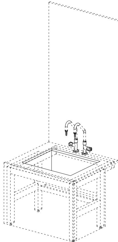
מבט איזומטרי
