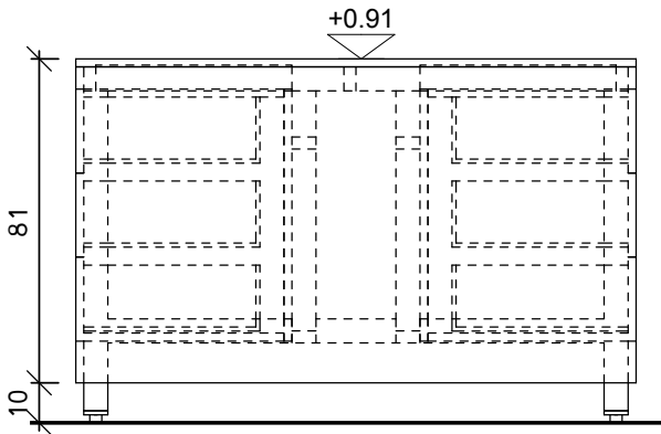
צד
