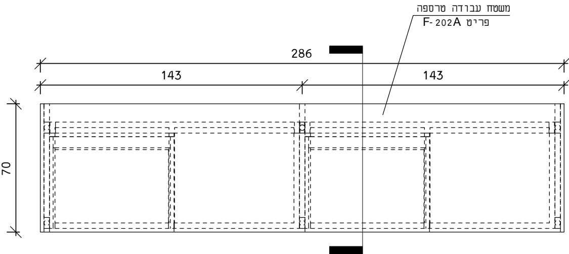
תכנית
