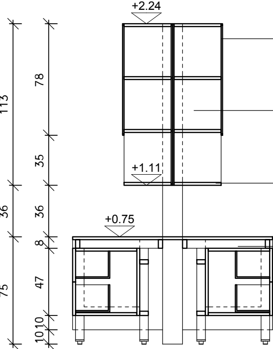
חזית
