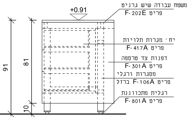
צד
