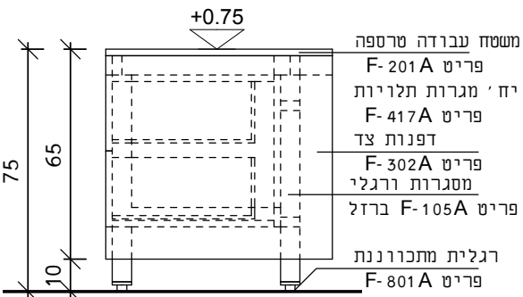
צד
