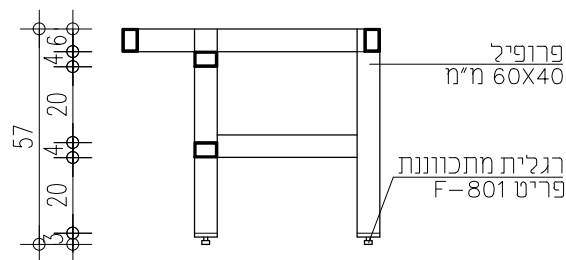
חותך 1:20
