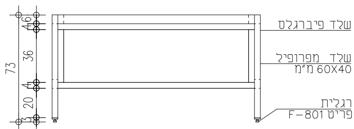
חזית 1:20
