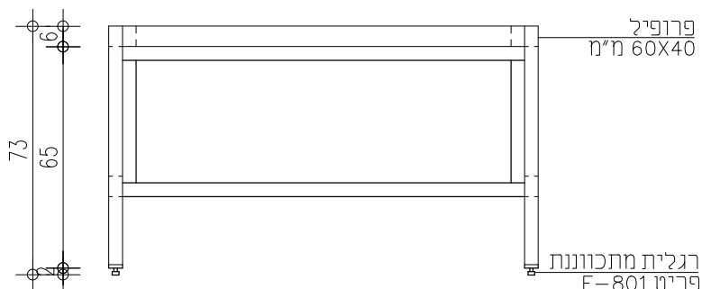
1:20 חתך
