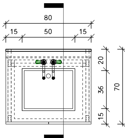
תכנית
