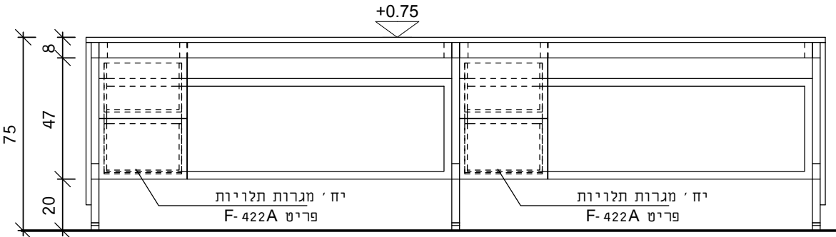
חזית
