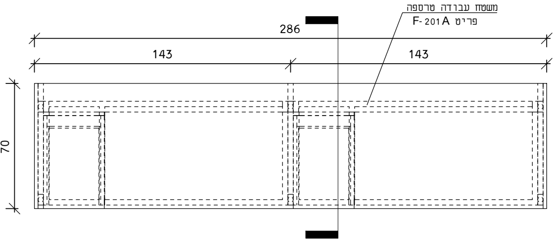
תכנית
