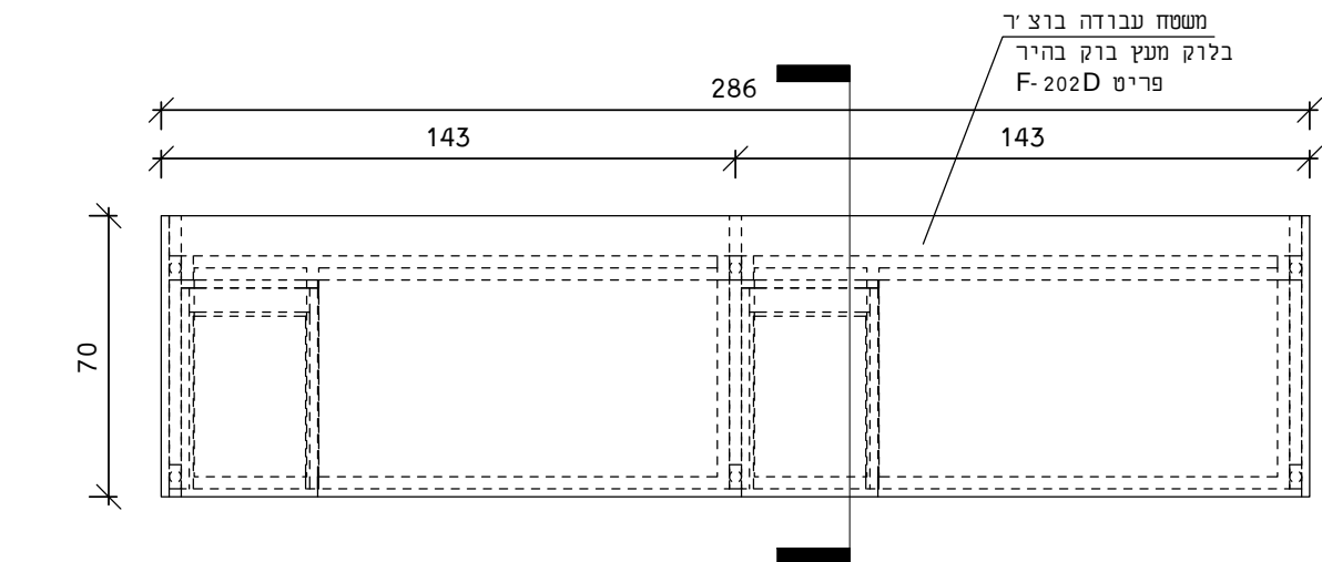
תכנית
