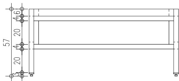
חזית 1:20
