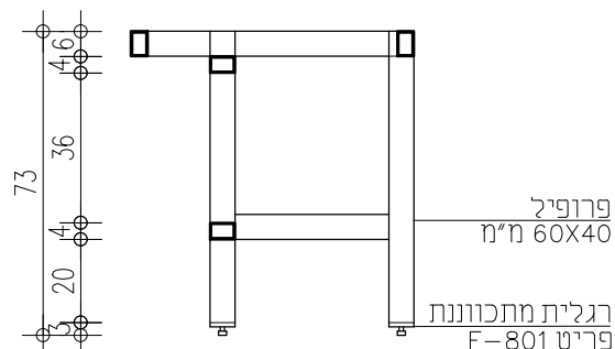
צדן 1:20
