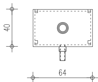
חזית צד 1:20
