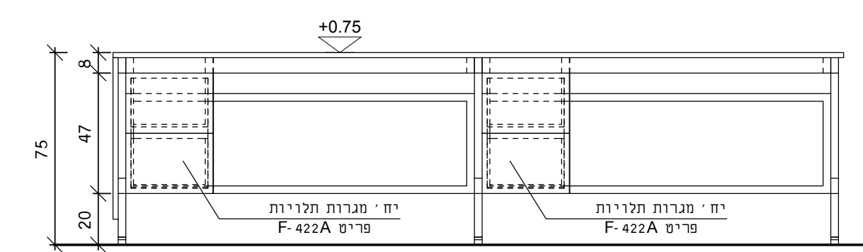
חזית
