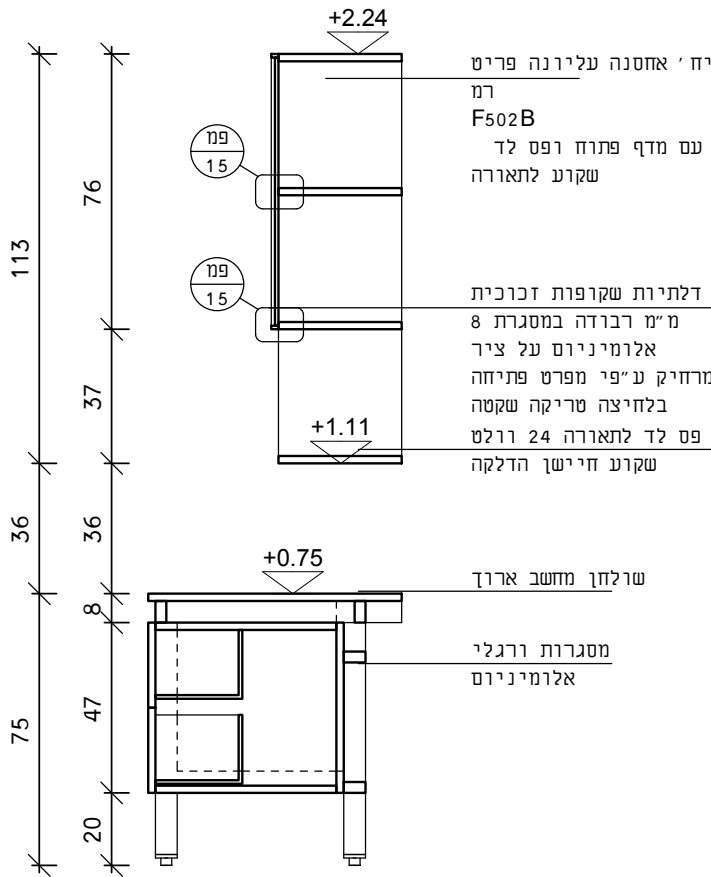
חזית
