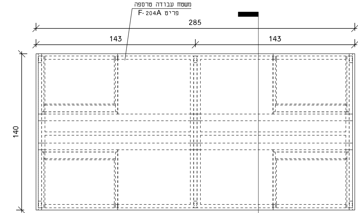
חזית
