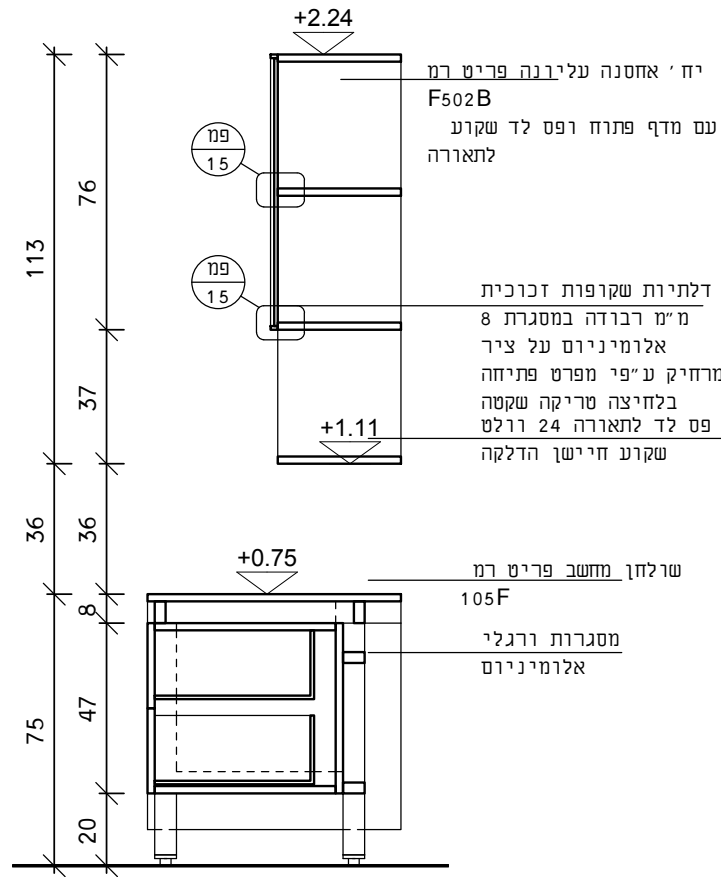
חזית
