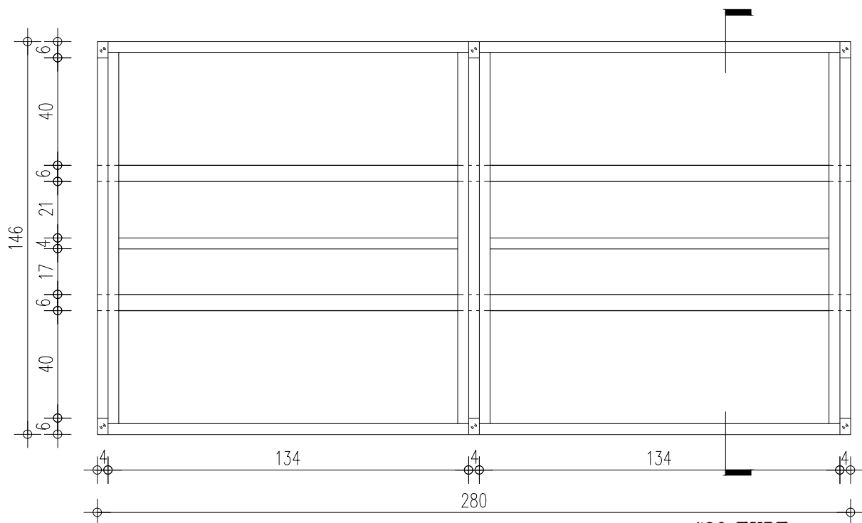
תכנית 1:20
