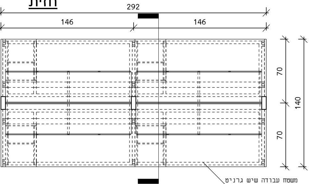
תכנית
