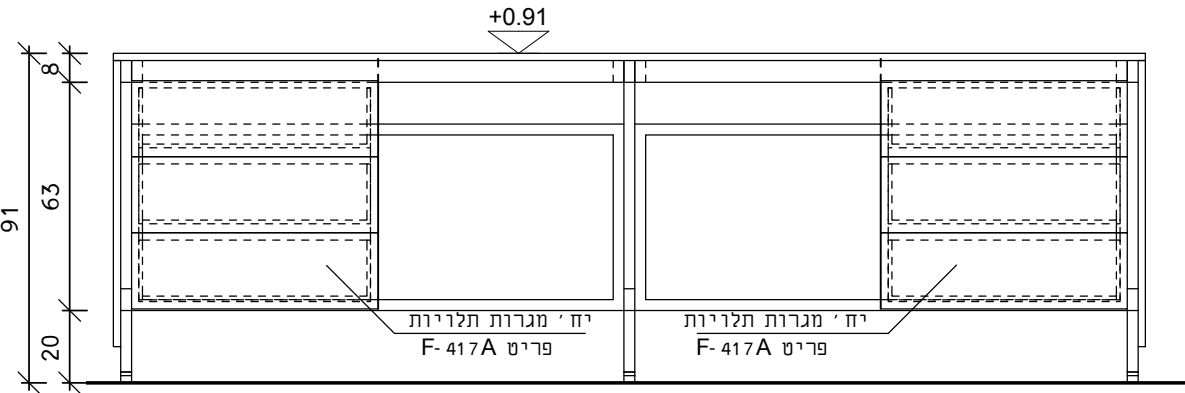
חזית
