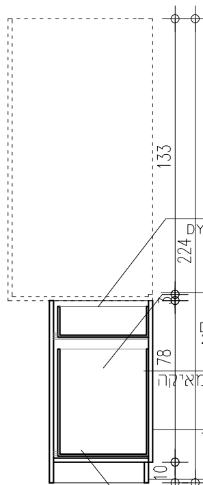
חתך 1:20
