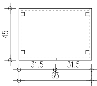
תכנית 1:20
