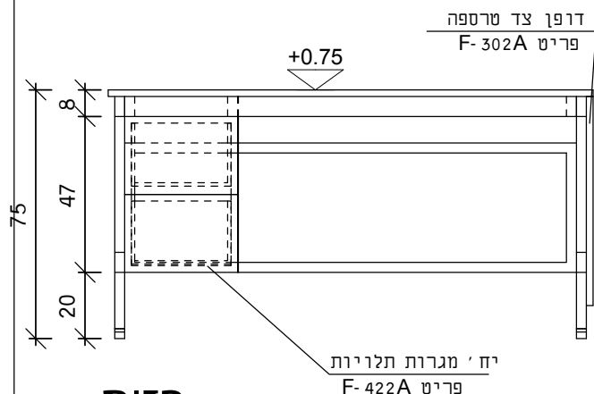
חזית
